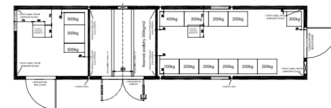
MODUL PRO TECHNOLOGIE TRAFOSTANIC 12 000 x 2 438 mm
