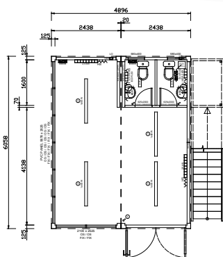
PŮDORYS 1.NP
