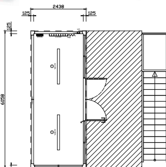
PŮDORYS 2.NP
